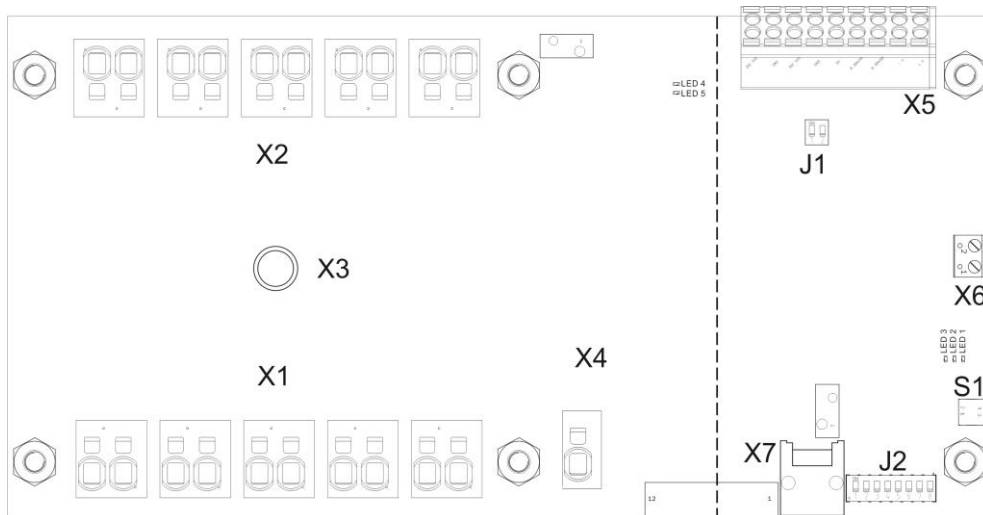
Abb. 5 Eingangsanschluss im KSM-Monitoring System
