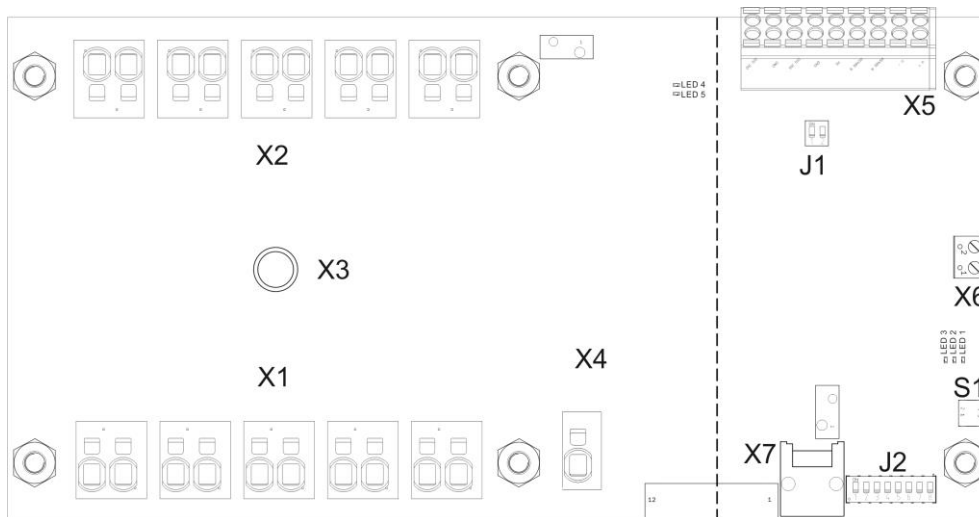
Abb. 6 Hauptleitungsanschluss im KSM-Monitoring System
