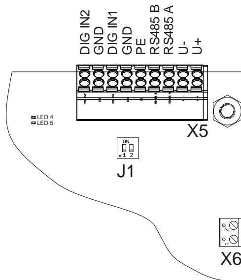
Abb. 3 Kommunikationsanschluss im KSM-Monitoring System
