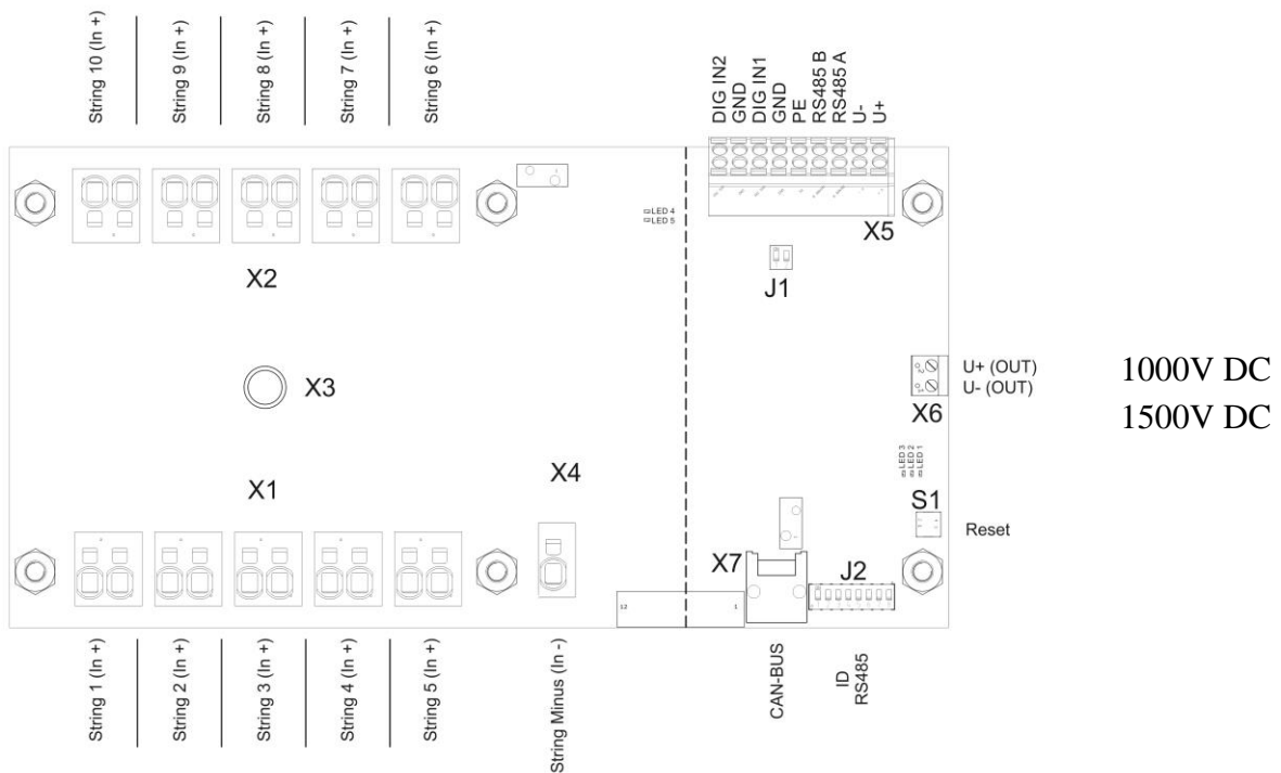
Abb. 1 ähnlich, Aufbau von der Ausführung des KSM-Monitoring System abhängig
