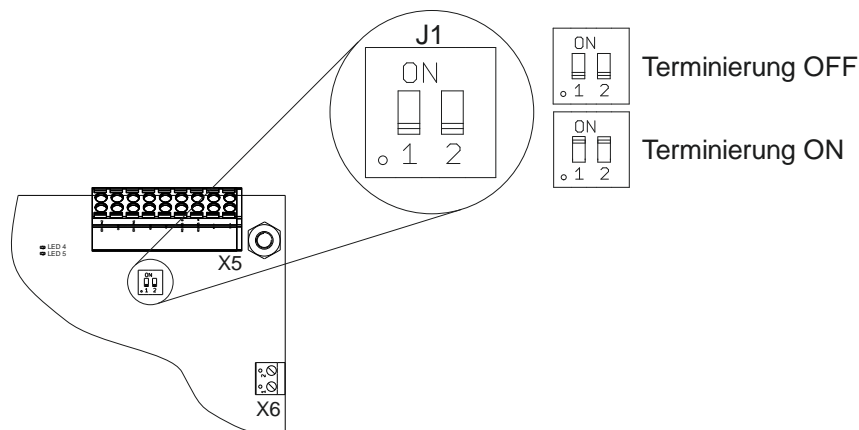
Abb. 8 Terminierung des KSM-Monitoring Systems
