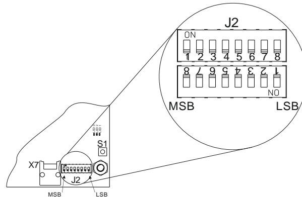
Abb. 9 Adresskodierschalter des KSM-Monitoring Systems
